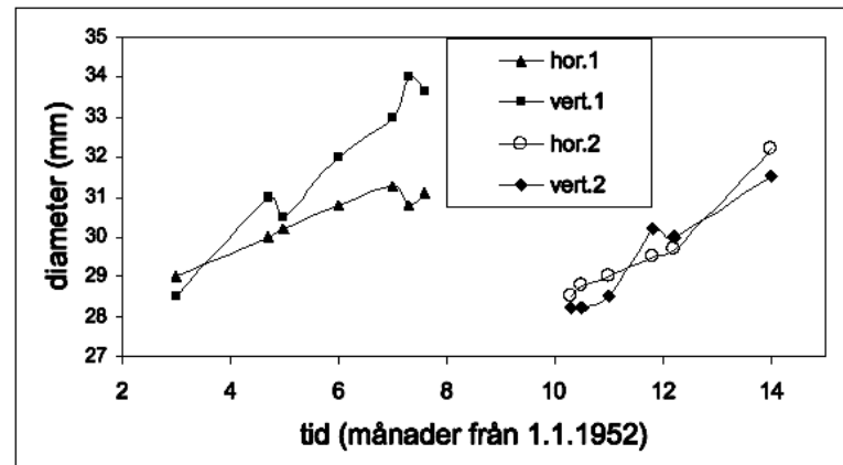
Figur 3. Stämpeldiameter som funktion av tillkomsttid för två gummistämplarna från Stockholm 19 (1952-3), mätt såväl horisontellt som vertikalt (genom streckstjärnan). Tre av dessa avtryck visas i Figur 4.
